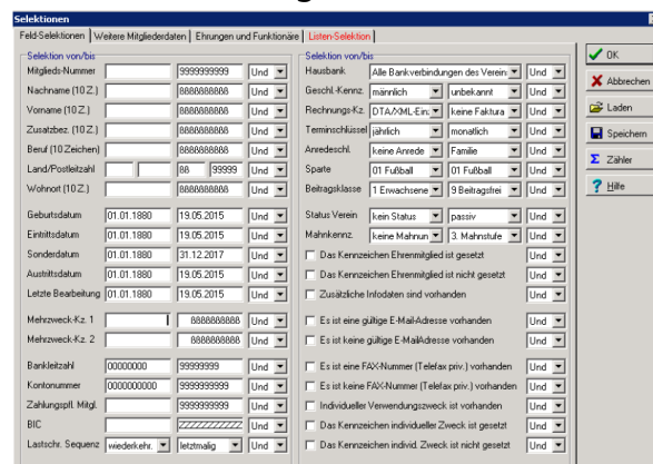
Abb. Selektionen - Reiter „Feld-Selektionen“
